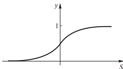
Рис. 4.11. Сигмоидная активационная функция y = f_{\sigma}(S)
