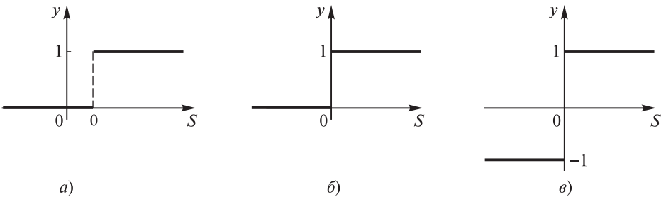
Рис. 4.3. Пороговые активационные функции нейрона, заданные формулами: a — (4.2); б — (4.4); в — (4.5)
