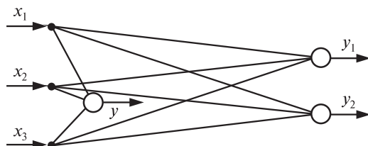
Рис. 7.2. Добавляется скрытый нейрон-кандидат, который своими синапсами подключается ко всем входным нейронам сети, а его аксон остается свободным
